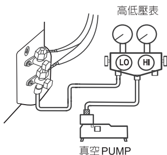
真空 PUMP
